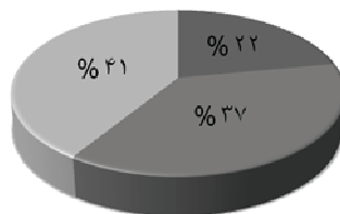
شکل ۳: تقسیمات نامساوی گردونه‌ی شانس
