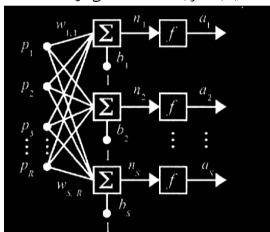
شکل ۶: شبکه‌ی عصبی تک‌لایه
